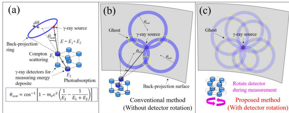
図 1 (a) コンプトンカメラの模式図 (b) 画像再構成法 (従来法) (c) 画像再構成法 (提案手法)
