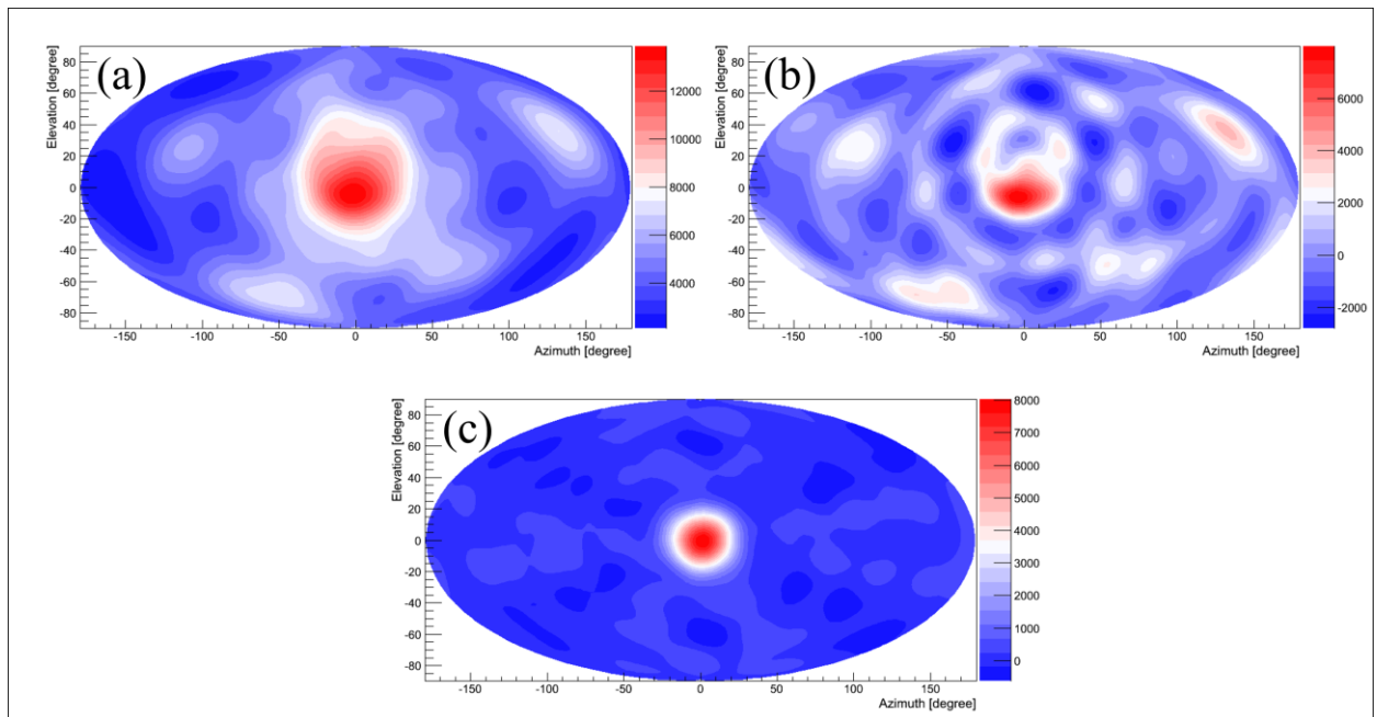
図 3 実験で得られた全方向 \gamma 線画像の例 (視野中心に ^{22}\text{Na} 密封線源 (放射能 : 1.6MBq、511keV \gamma 線放出)、検出器-線源間距離 1m、エイトフ図法で表示 (左右が水平方向、上下が垂直方向を表す))
