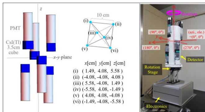
図 2 今回の実証試験に用いたコンプトンカメラの模式図と外観写真
