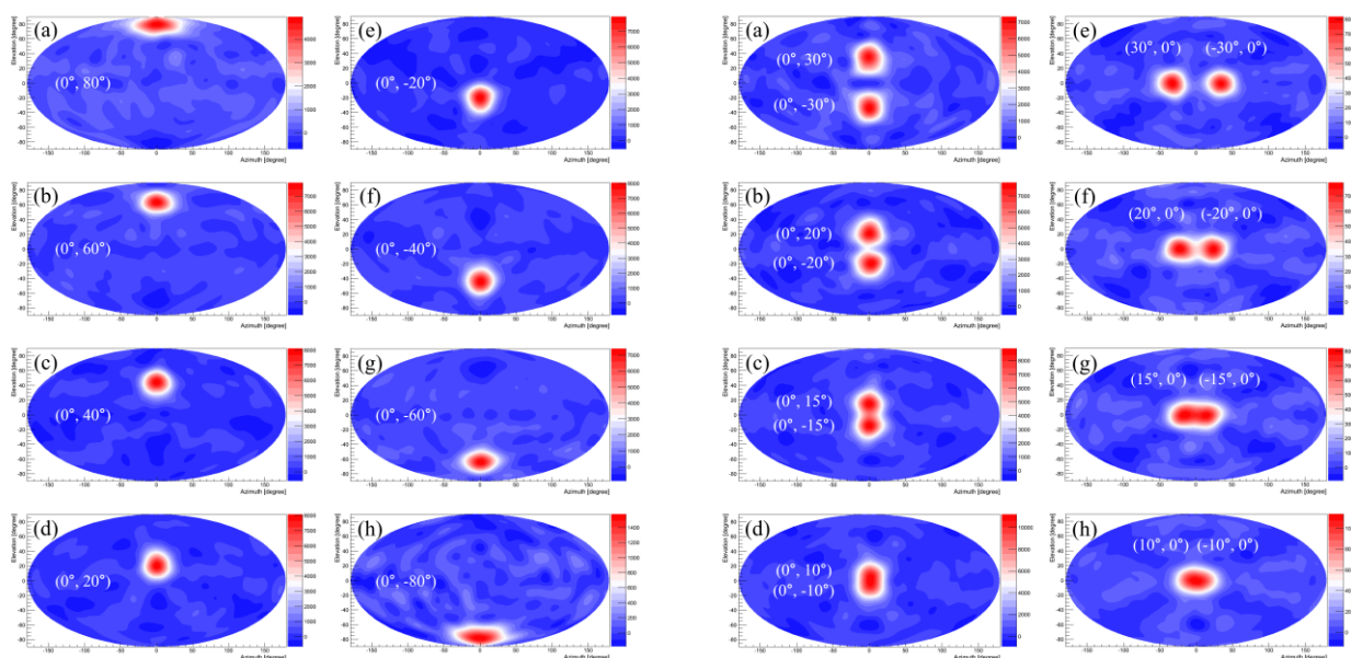
図4 \gamma 線源がさまざまな方向にある場合の結果 ( ^{22}\text{Na} 密封線源、検出器-線源間距離 1m、画像フィルタあり、回転あり)
