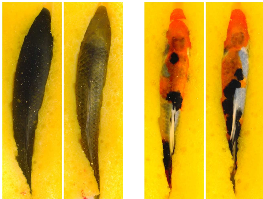
【画像2】 黒水槽と白水槽に馴致したマゴイ（左）と大正三色（右）
